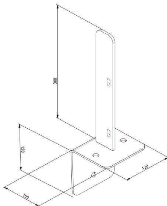
PLATINE L OU ÉQUERRE
