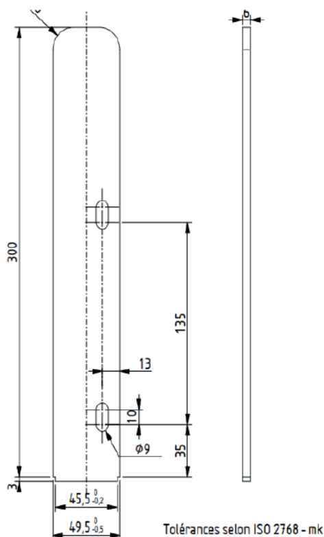
PLATINE MANCHON OU OPTION SOUDÉ
